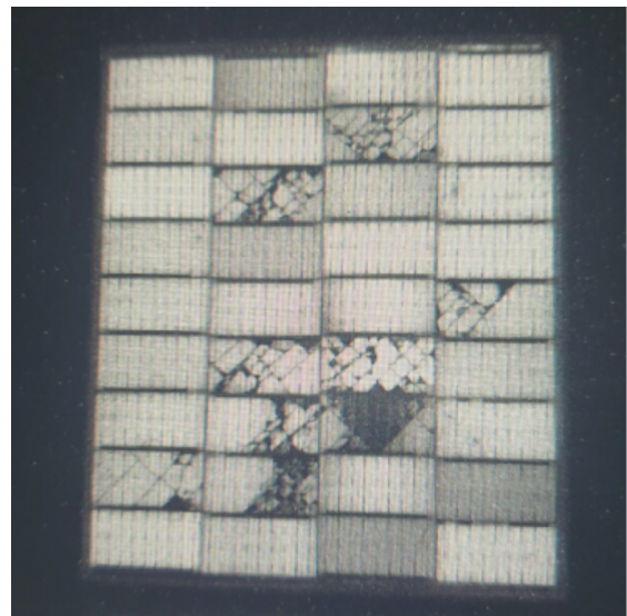
수축팽창에 의해 손상된 것으로 추정되는, 태양광 패널
